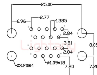
PCB布局 (PCB Layout)
